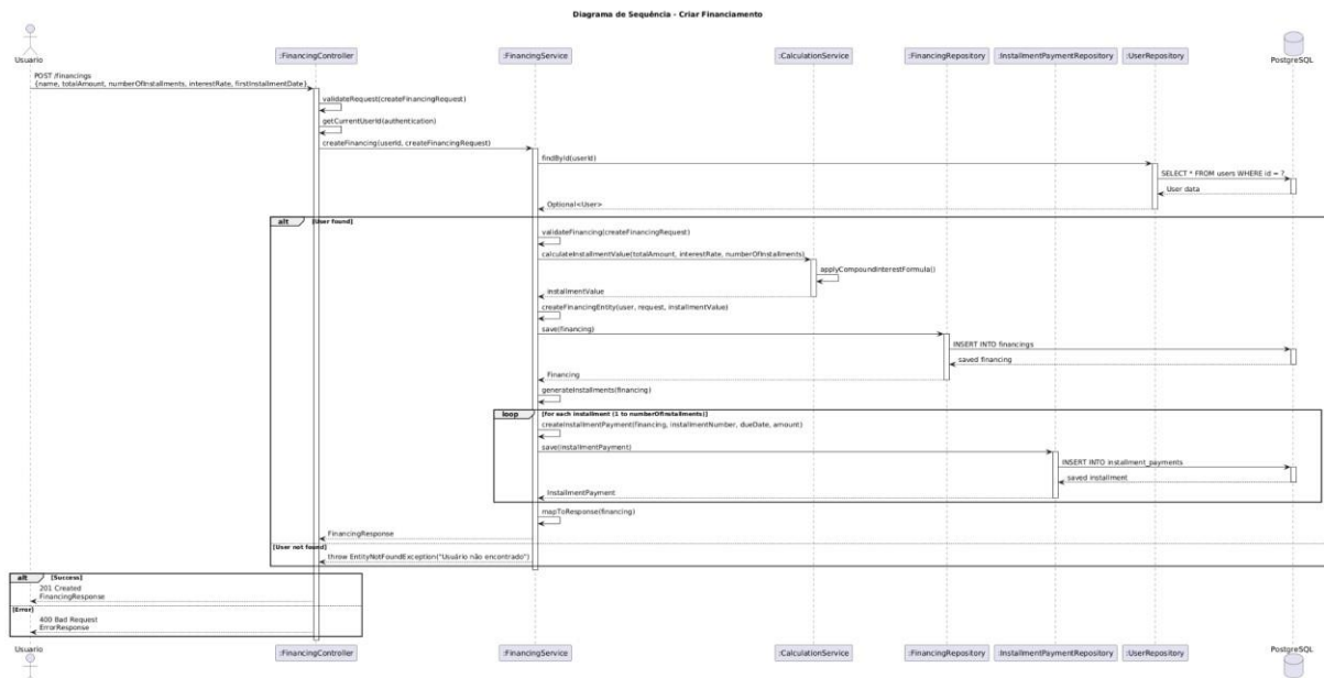
Figura 5: Fluxo de mensagens para a criação de um novo financiamento.
